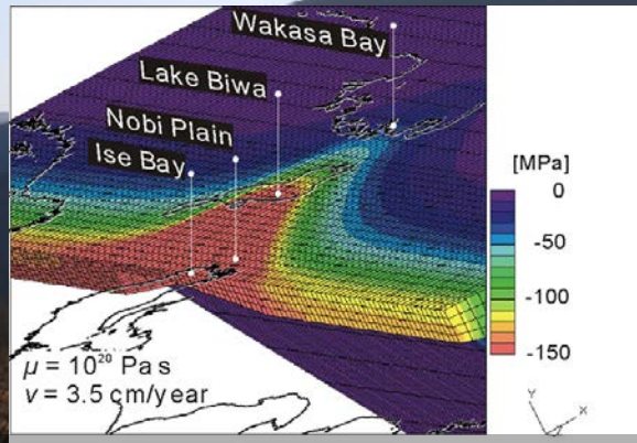
フィリピン海プレートの形状を考慮したマントル流シミュレーション(圧力効果) (Kudo & Yamaoka, 2003)
